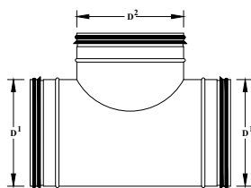
E6271 90° TEE
