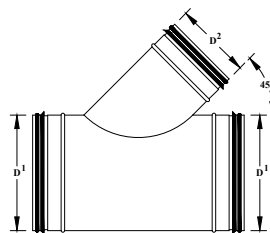
E6276 45° LATERAL
