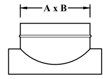
FO6307 90° SADDLE TAP
