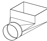
243 90° ANGLE BOOT
