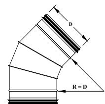
E6121 45° ELBOW 14" - 36" 3 Piece Gorelock
