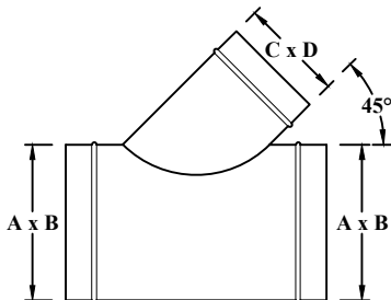
FO6276 45° LATERAL
