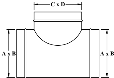
FO6271 90° TEE
