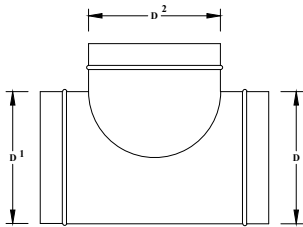
SP6271 90° TEE
