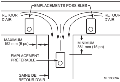
Fig. 3. Emplacements possibles pour installation sur une gaine.
