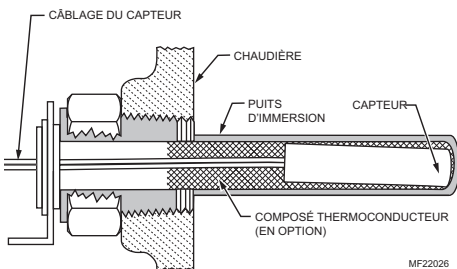
Fig. 5. Installation du capteur de rechange.
