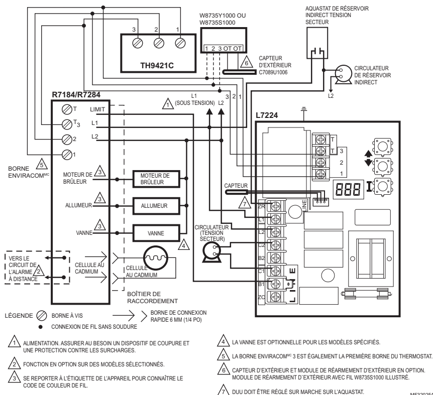
Fig. 12. Système à zone unique L7224U avec circulateur, réservoir d'eau indirect et thermostat EnviraCOM MC .
