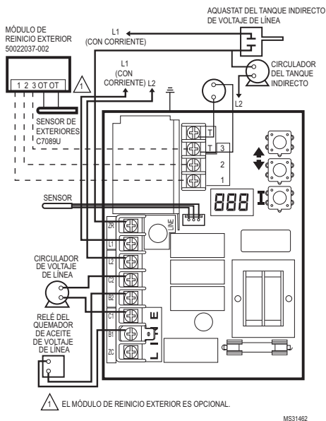
Fig. 9. L7224U de una sola zona de calor con tanque de agua indirecto y circuladores. Módulo de inicio exterior opcional.
