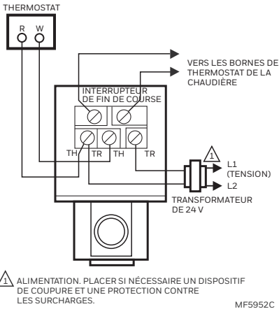
Fig. 5. Câblage typique de la vanne V8043F.
